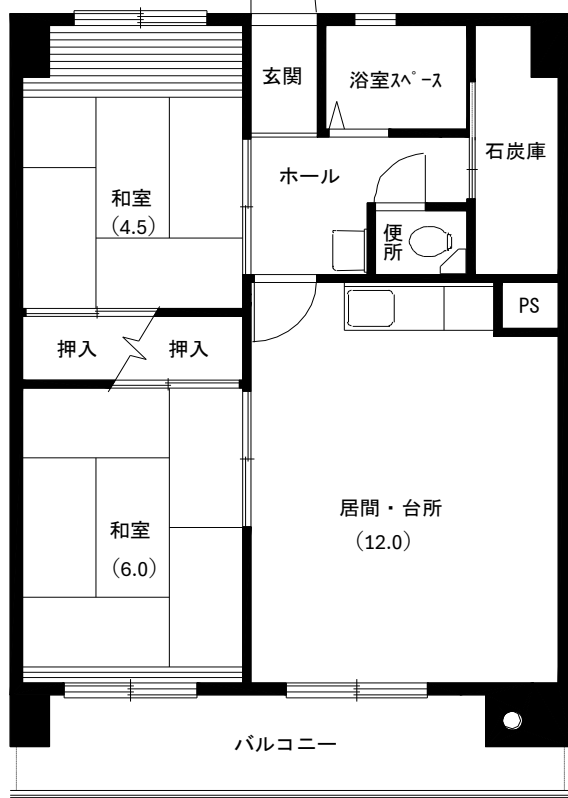
平面図
